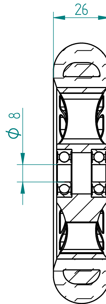
SECTION A-A
